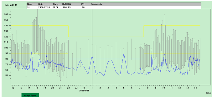
Abbildung 6.10.2 Trenddiagramm mit gepunkteter Linie
